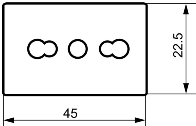
Disegno quotato
