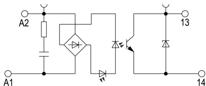
Schaltymbol
