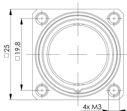
Disegno quotato
