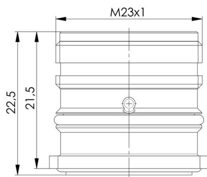
Disegno quotato
