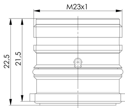
Disegno quotato
