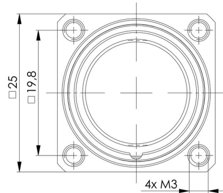
Disegno quotato
