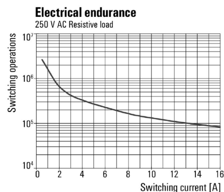
Elektromos élettartam
