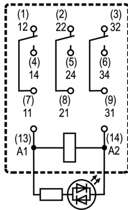
Csapok alulnézetben
