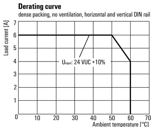
Visszaszabályozási görbe
