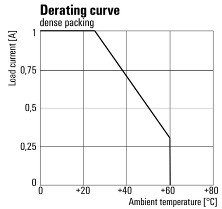
Visszaszabályozási görbe
