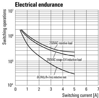
Elektromos élettartam
