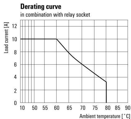
Visszaszabályozási görbe
