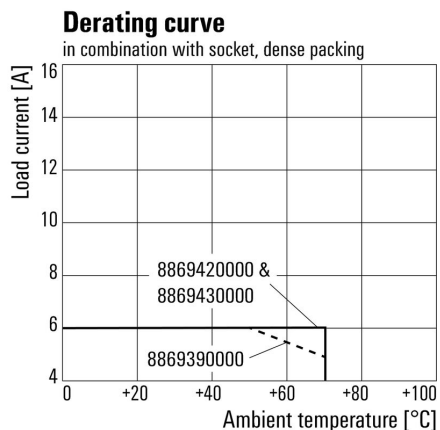
Visszaszabályozási görbe Relay in combination with base
