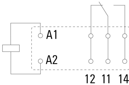
Vue des broches par dessus
