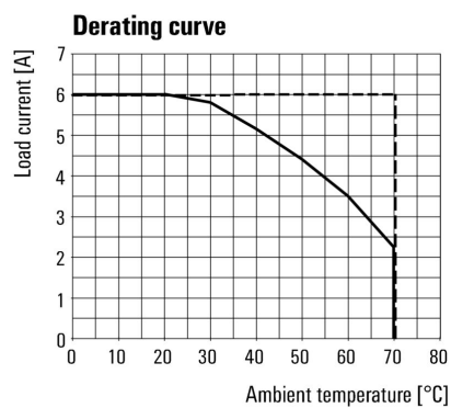
Courbe de dérating
