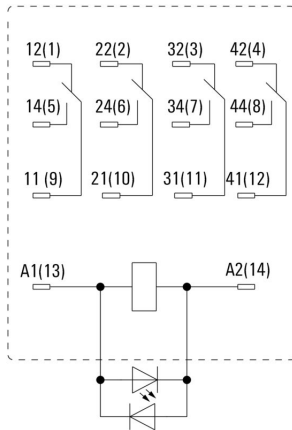
Vue des broches par dessous
