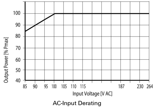
Courbe de dérating
