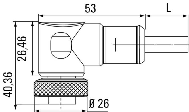
Dessin coté
