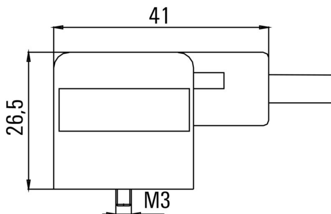
Dessin coté
