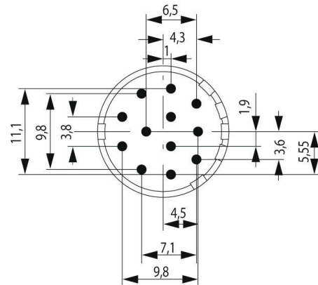
Dessin coté
