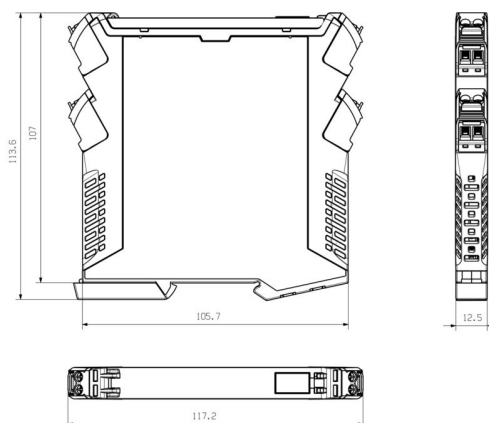
Dessin coté
