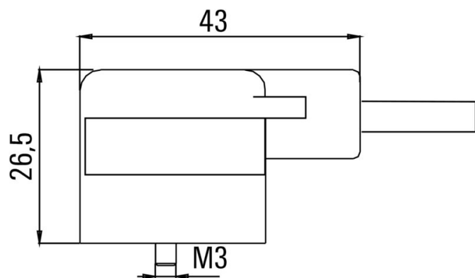
Dibujo acotado
