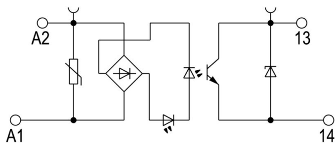
Schaltymbol
