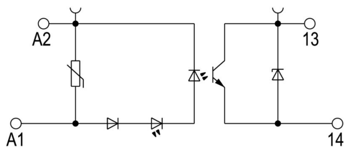
Schaltssymbol
