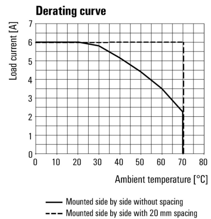
Curva de deriva
