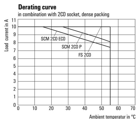
Curva de deriva Relé combinado con base
