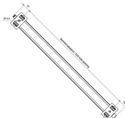
Dibujo acotado
