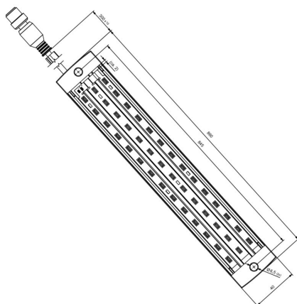
Dibujo acotado
