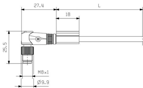
Dibujo acotado
