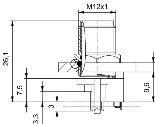
Dibujo acotado
