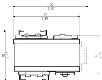
Dibujo acotado
