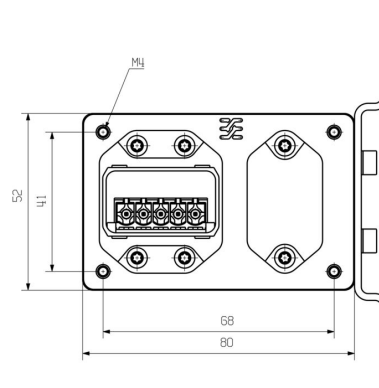
Dibujo acotado
