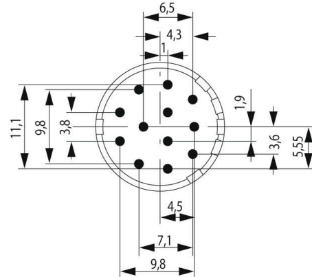
Dibujo acotado
