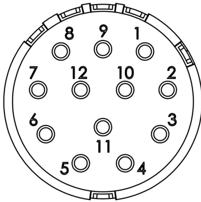
Dibujo acotado
