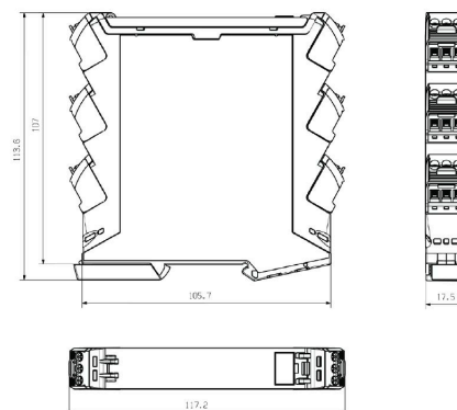
Dibujo acotado
