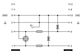
Complete module direct grounding Komplettschaltmodul direkte Erdung
