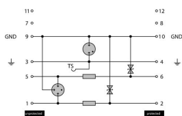
Complete module indirect grounding Komplettschaltmodul indirekte Erdung
