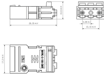
Steckverbinder Bauform 1 Connector type 1
