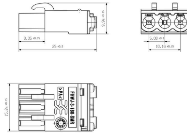
Steckverbinder Bauform 3 Connector type 3
