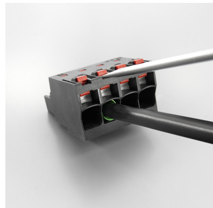
Quick wiring
