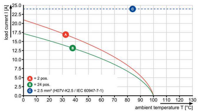
BLZP 5.08/.. /180 - SL 5.08/.. /90
