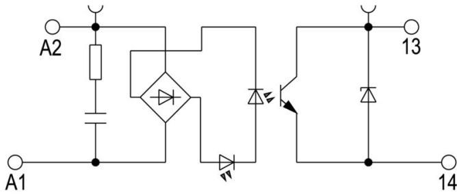
Schaltssymbol
