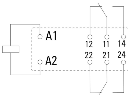
Ansicht auf Pins von unten
