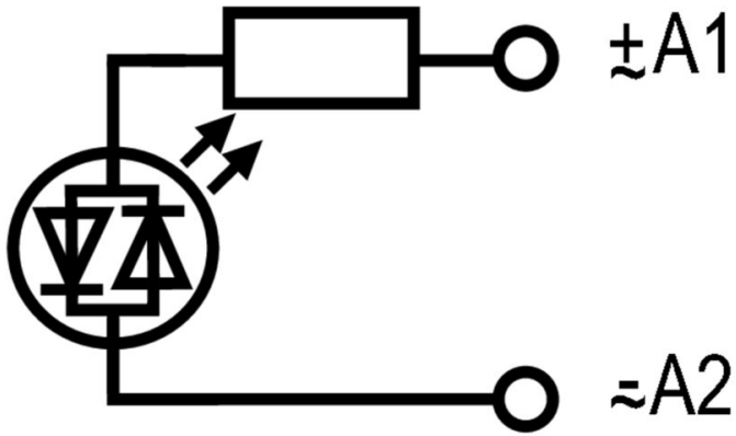
Schaltbild
