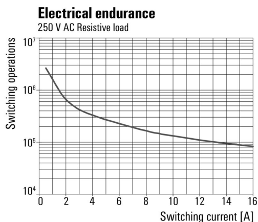
Elektrische Lebensdauer
