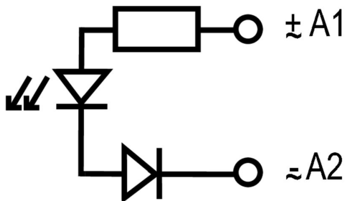
Schaltbild
