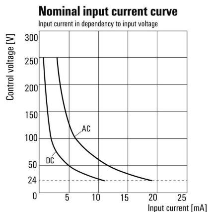
Eingangsstrom ist abhängig von der Eingangsspannung
