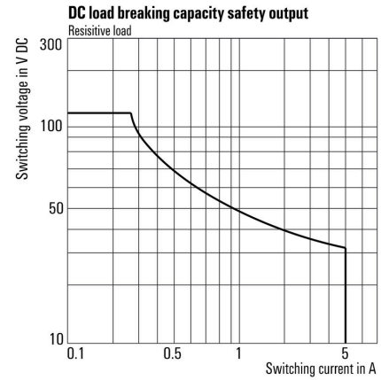
Lastgrenzkurve DC
