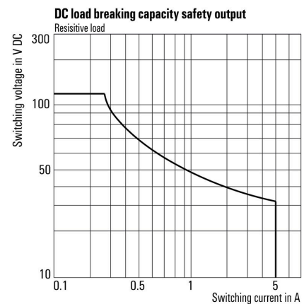
Lastgrenzkurve DC
