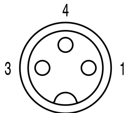
Socket
