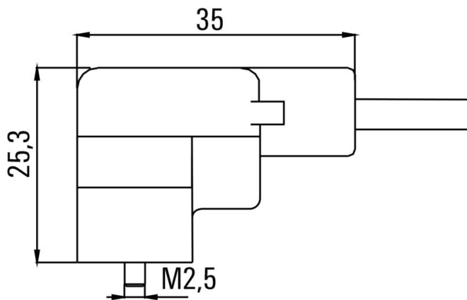
Maßzeichnung
