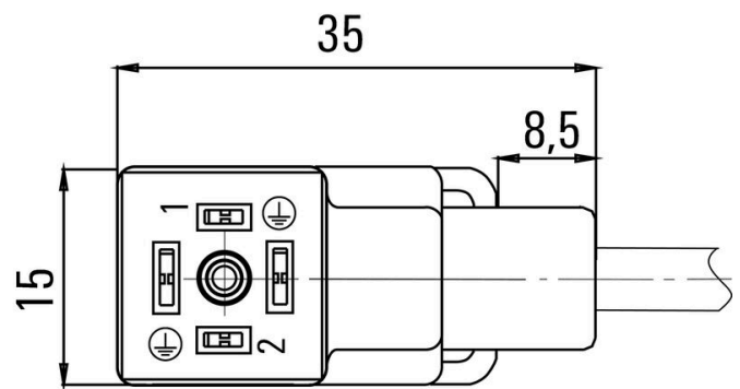
Polbild
