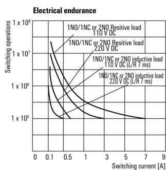
Elektrische Lebensdauer
