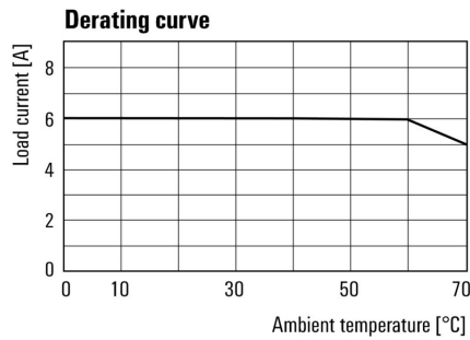
Lastgrenzkurve DC
