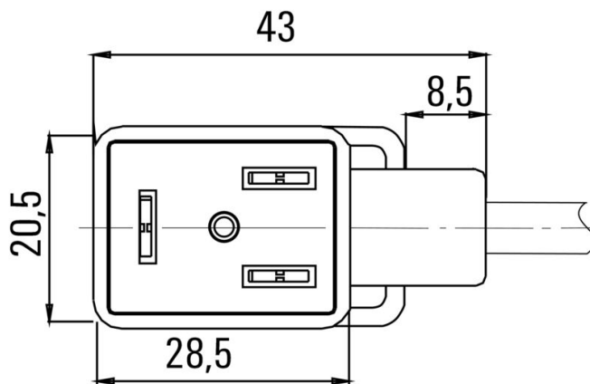
Schéma pólů
