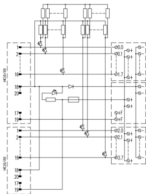
Elektrické schéma odpovídá verzi s LED.
